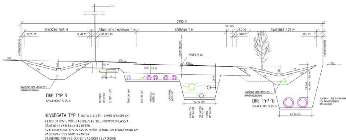
Exempel på gatussektion ur PM Gata, VA och övriga ledningar.
