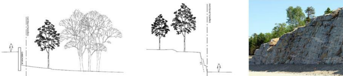
Exempel gabionmur mot fyllnad av kvartersmark och exempel på trappad bergskärning 5:1 med variation i slänfotens avstånd till asfaltytan. Bergskärningar ska utföras med skonsam sprängning.
