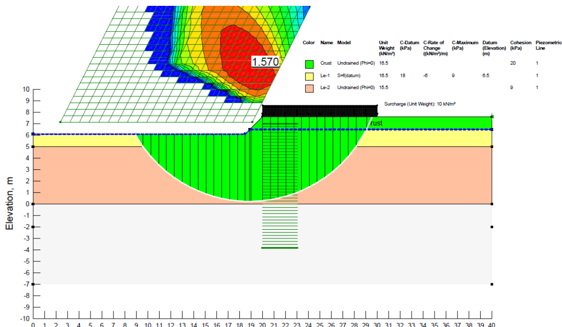
Figur 8.2 Stabilitet vid 1,5m djup schakt
