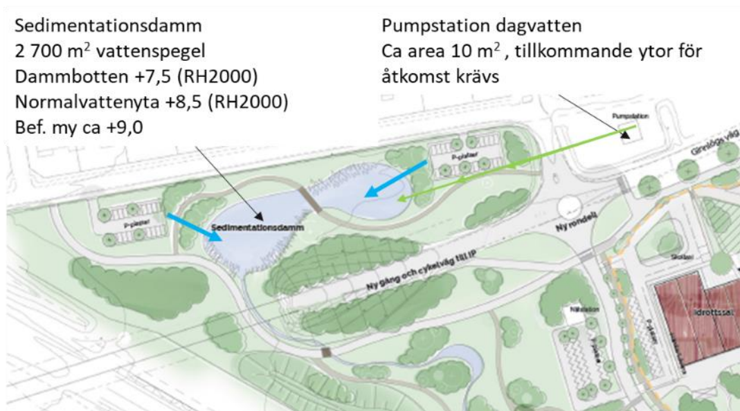
Figur 7. Föreslagen sedimentationsdamm för rening av dagvatten från avrinningsområdet uppströms. Ljusblå pilar återger förslag på höjdsättning av planerade parkeringsytor för rening i sedimentationsdammen.
