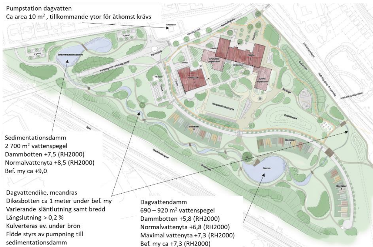
Figur 6. Föreslagen placering och dimensioner för dagvattendammar och diken.
