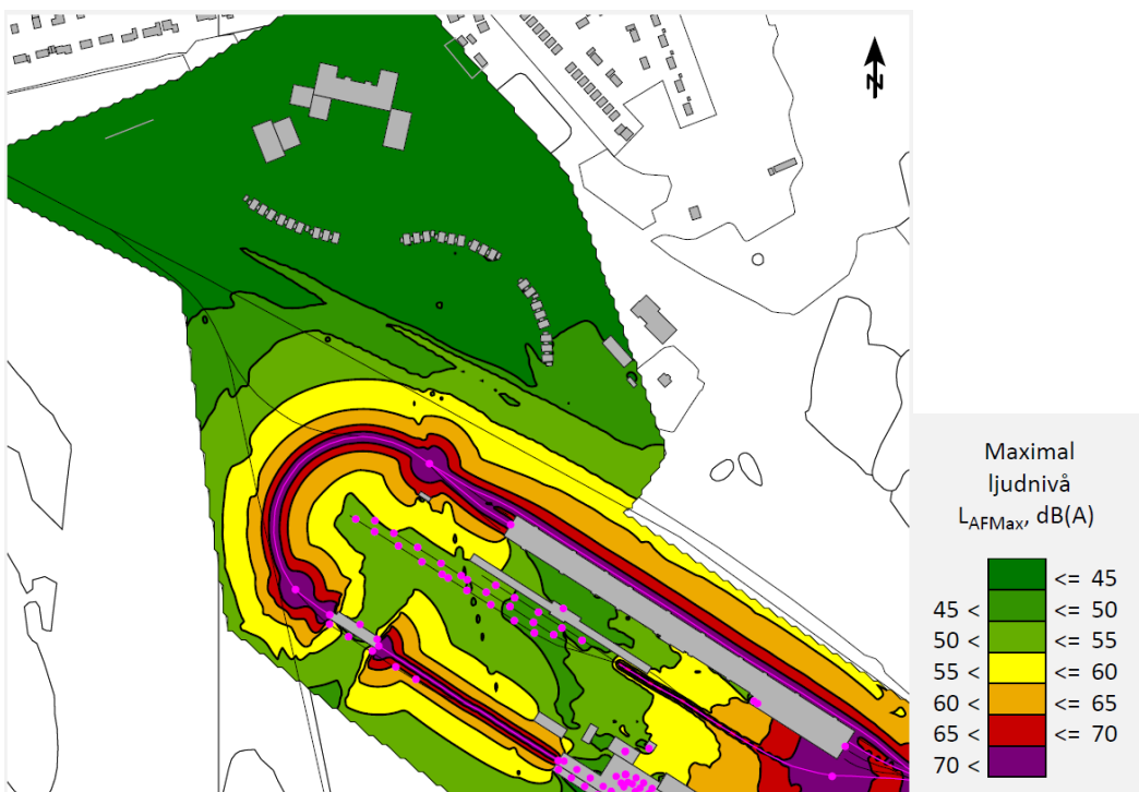
Bullerspridningskarta maximal ljudnivå industri. Beräkning inkluderar 5m skärning mot järnvägen och 3m skärning mot Enköpingsvägen. Bild: Brekke & Strand
