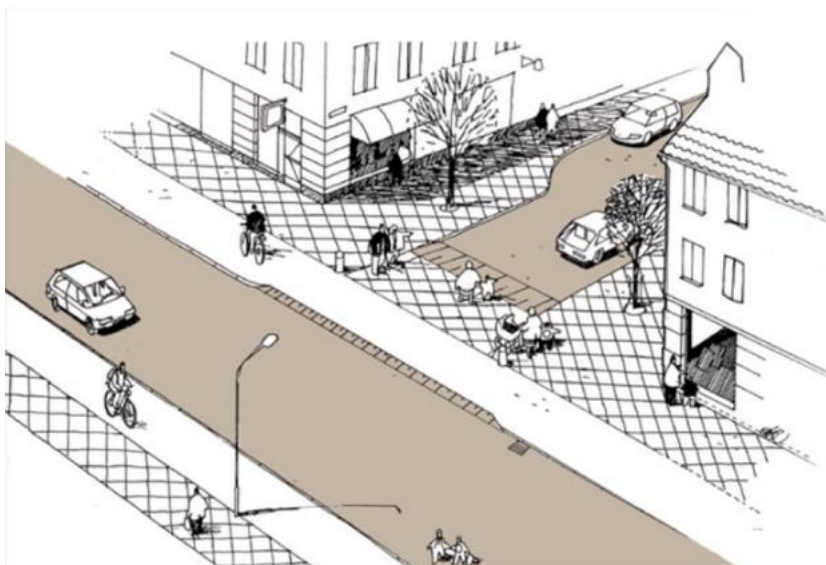
Typskiss över genomgående gång- och cykelbana-bana över anslutande lokalgata (Åtgärds katalog för säker trafik i tätort, Trafikverket, 2009)
