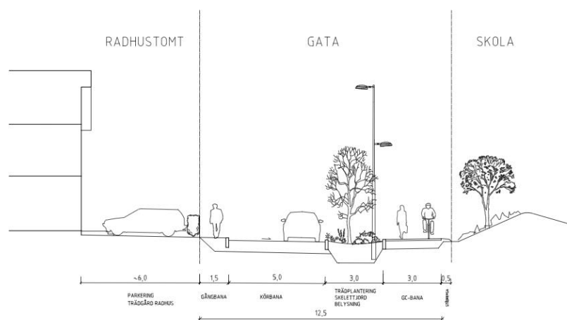
Gatusektion över lokalgatan, gång- och cykelbanan samt förgårdsmarken vid bostäderna av Topia
