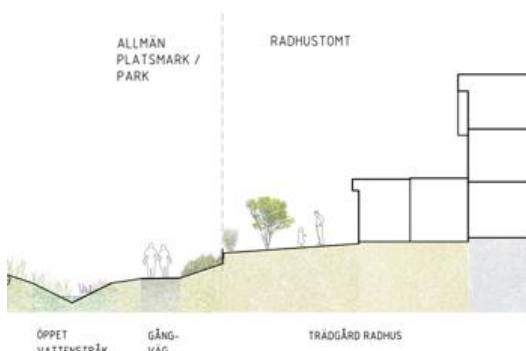
Sektion med höjdskillnaden mellan bostadsfastighet och park. Illustration av Topia.
