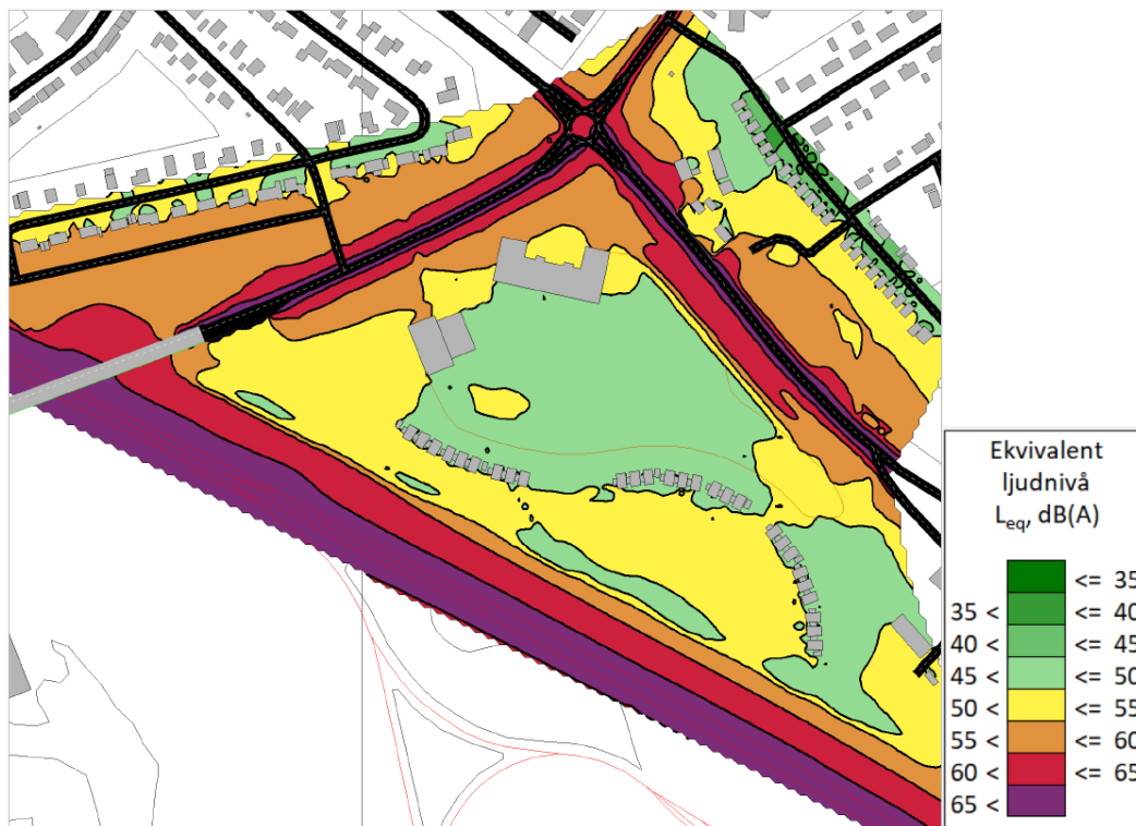
Bullerspridningskarta ekvivalent ljudnivå väg & järnväg. Beräkning inkluderar 5m skärmning mot järnvägen och 3m skärmning mot Enköpingsvägen. Bild: Brekke & Strand
