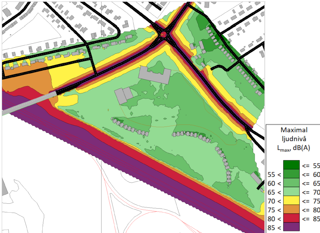
Bullerspridningskarta maximal ljudnivå väg & järnväg. Beräkning inkluderar 5m skärmning mot järnvägen och 3m skärmning mot Enköpingsvägen. Bild: Brekke & Strand
