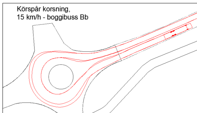
Körspår genom cirkulation med VGU-typfordon Boggibuss Bb med hastighet 15 km/h från Trivector
