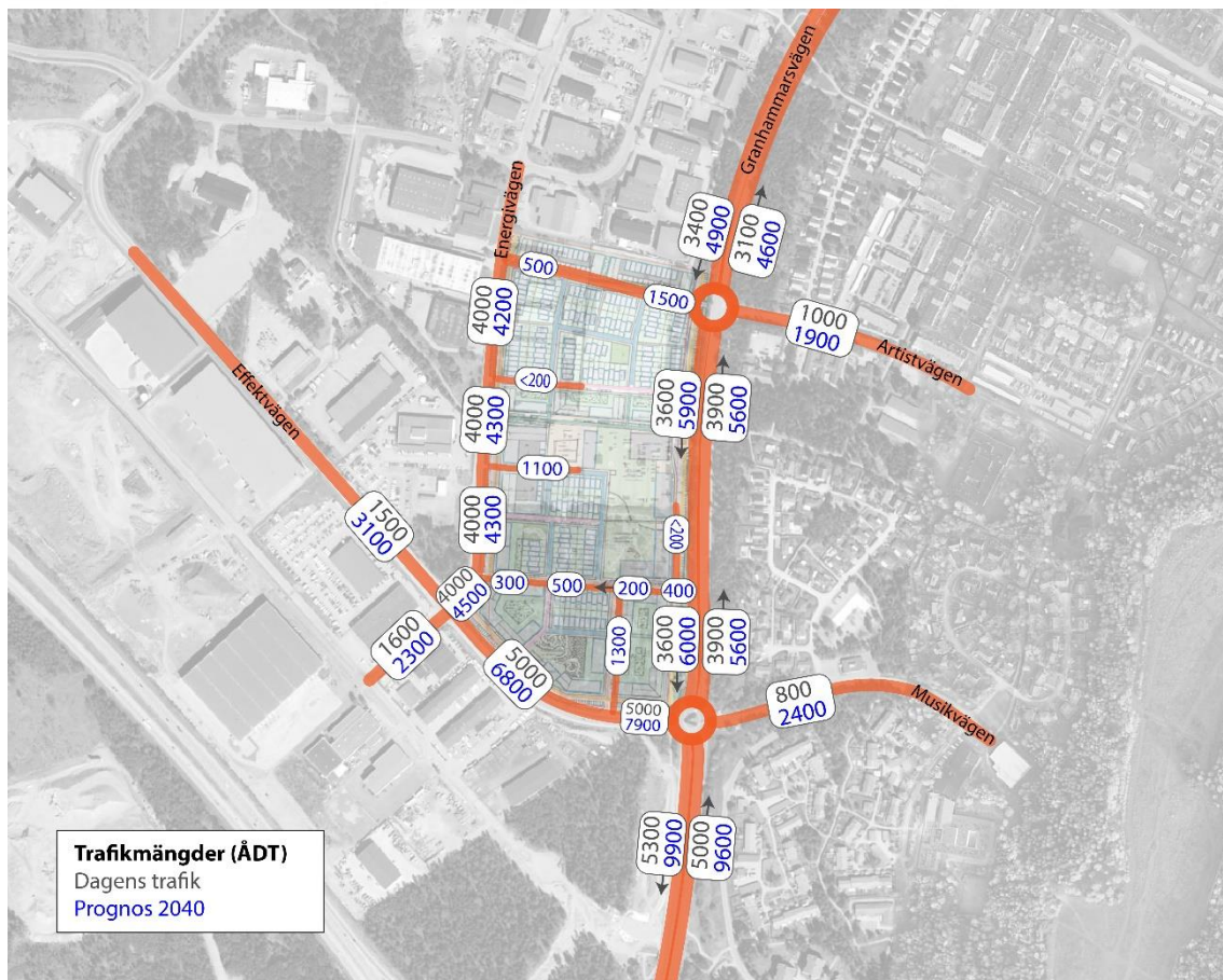
Figur 11. Trafikmängder ÅDT, dagens trafik och prognos 2040.
