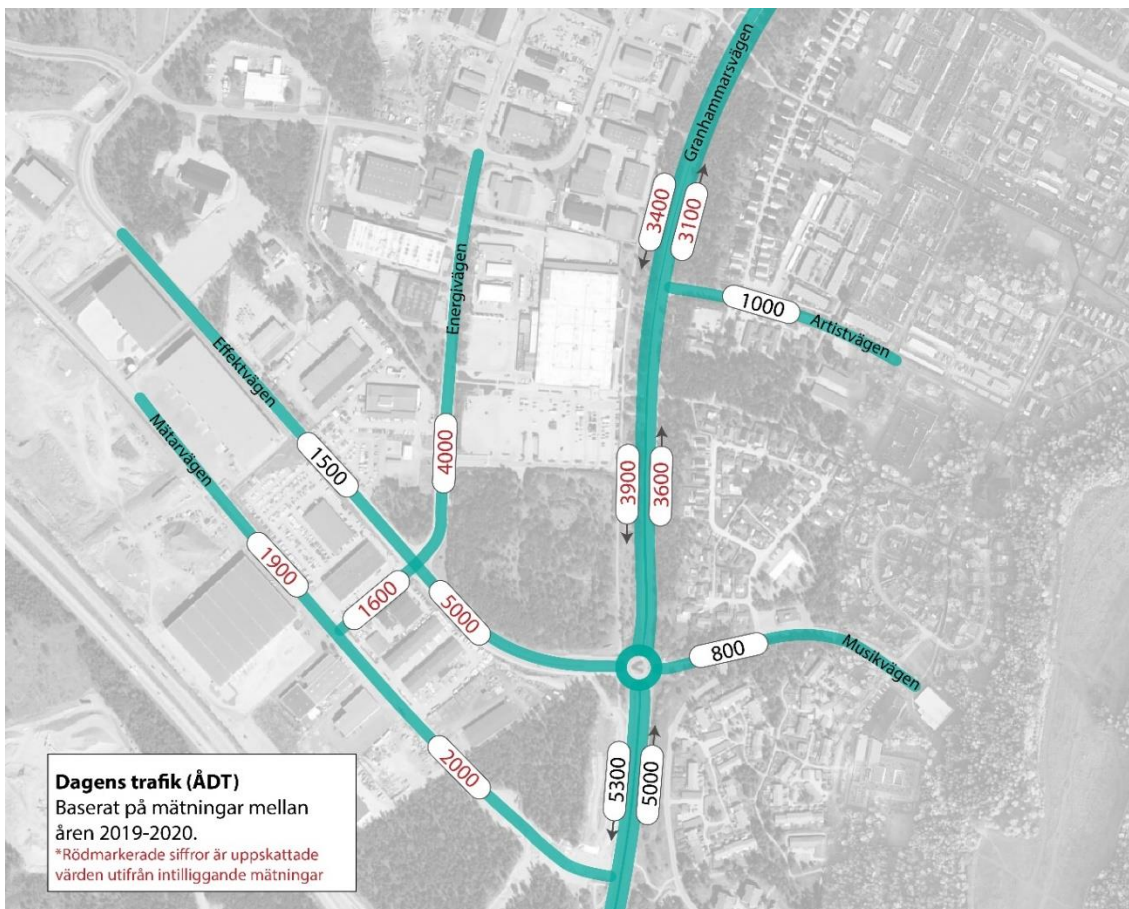
Figur 7. Dagens trafikflöden (ÅDT).
