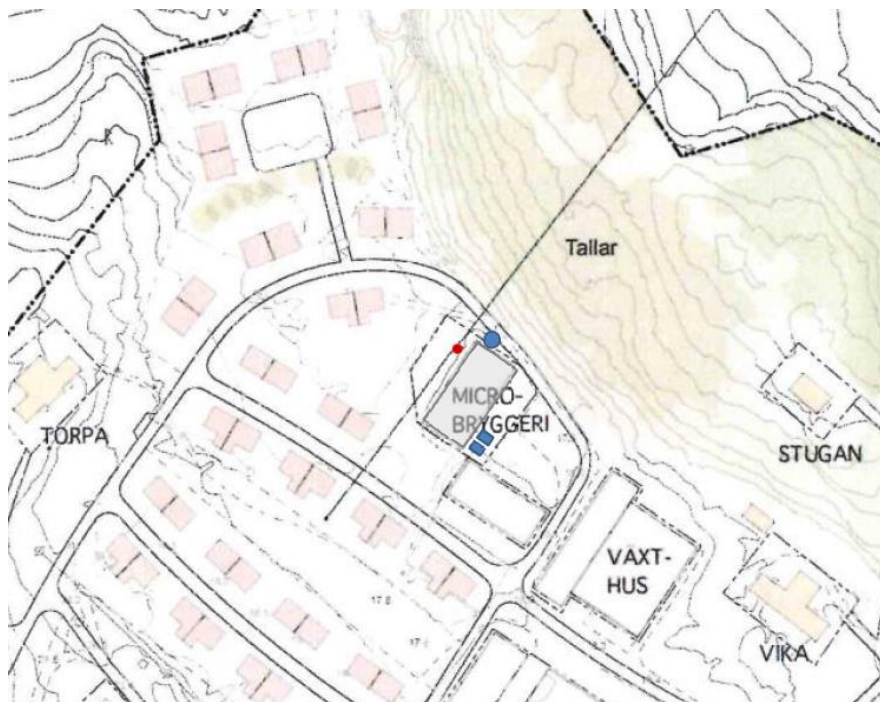
Figur 6.8. Intill mikrobryggeriet finns fyra externa ljudkällor; en ångpanna väster om byggnaden (röd markering), en frånluftsvärmepump vid den norra fasaden (blå cirkel), samt två kylmedelskylare öster om byggnaden (blåa kvadrater). Bildkälla: Mätning av ljudnivåer från bryggeri 27 .
