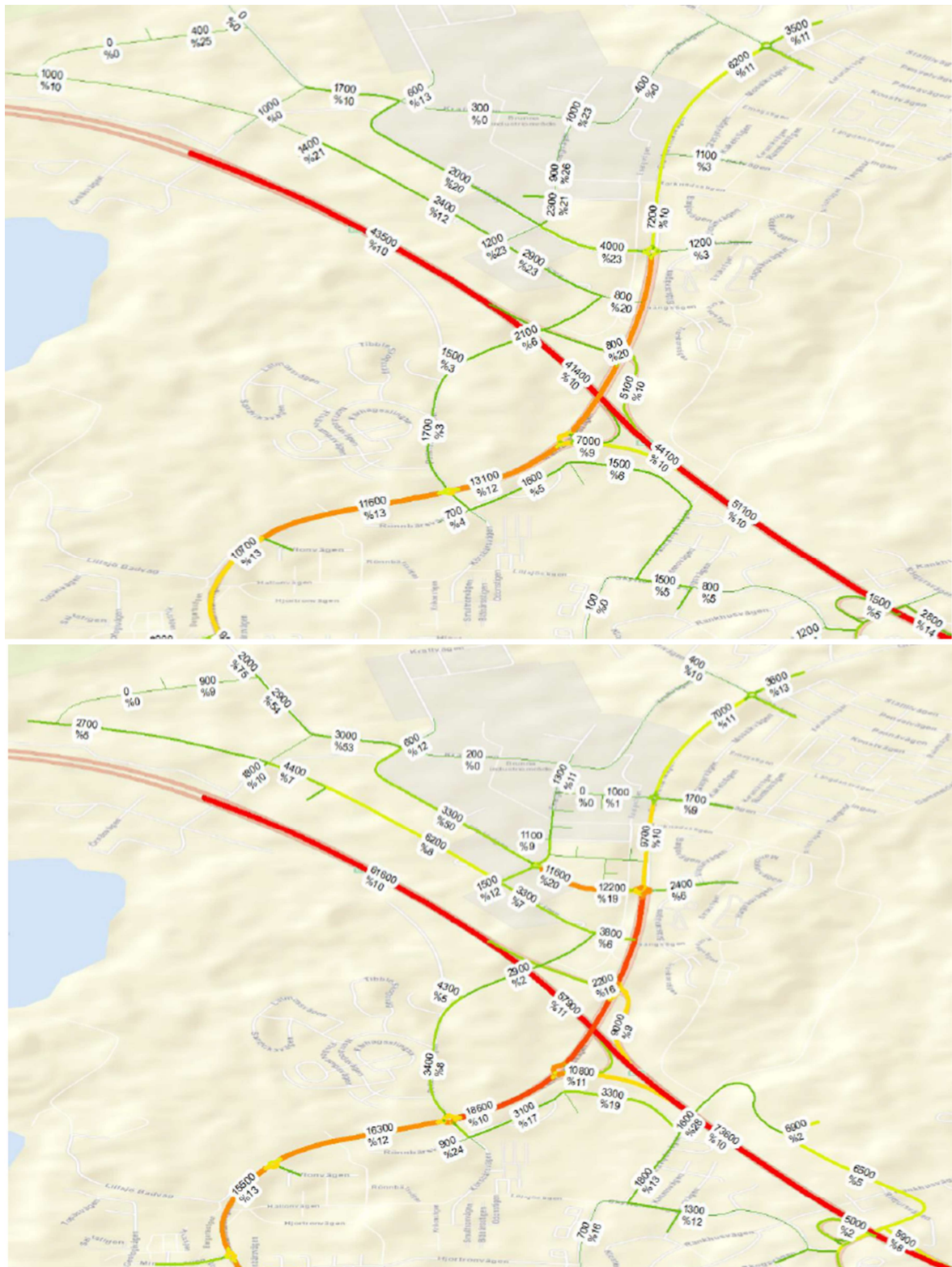
Figur 12 a och b Dagens trafikflöden ÅDT (överst) och prognosticerade trafikflöden ÅDT för 2040 (nederst). Procenttal visar andel tung trafik. (Afrý 2021-03-31)
